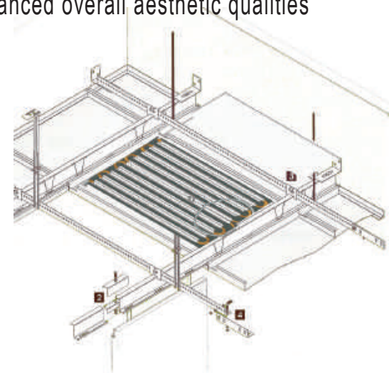
拼装式模块化辐射金属吊顶板 Komfo-Blitz-G 系列
